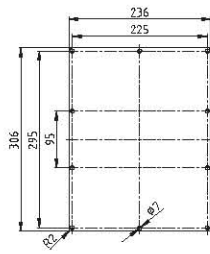
BAK 13 - ST 13 / AL 13 铜: 4 mm 厚; 2,2 kg 铝: 5 mm 厚; 1,0 kg
