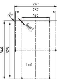
BAK 10 - ST 10 铜: 3 mm 厚; 1,9 kg
