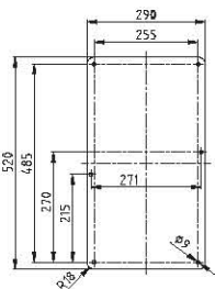
BAK 20 - ST 20 / AL 20 铜: 5 mm 厚; 5,8 kg 铝: 5 mm 厚; 2,0 kg
