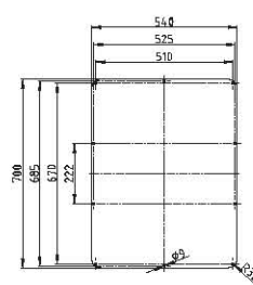
BAK 100 - ST 100 / AL 100 铜: 6mm厚; 17,8 kg 铝: 8 mm 厚; 8,2 kg
