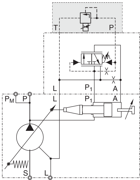
原理图, PVACPP*
