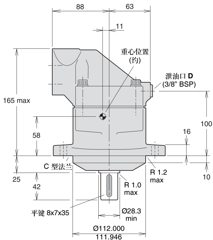
C 型安装法兰
