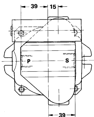
A向视图
