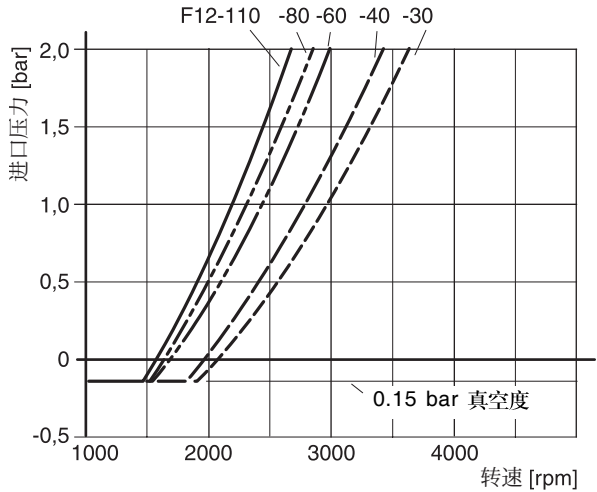
图3.所需的马达最低进口压力(F12-M)
