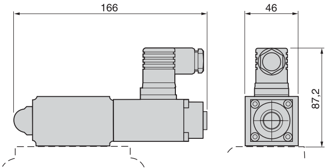
尺寸, PVACPP*
