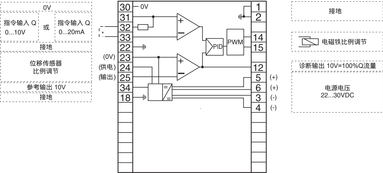
线路图
