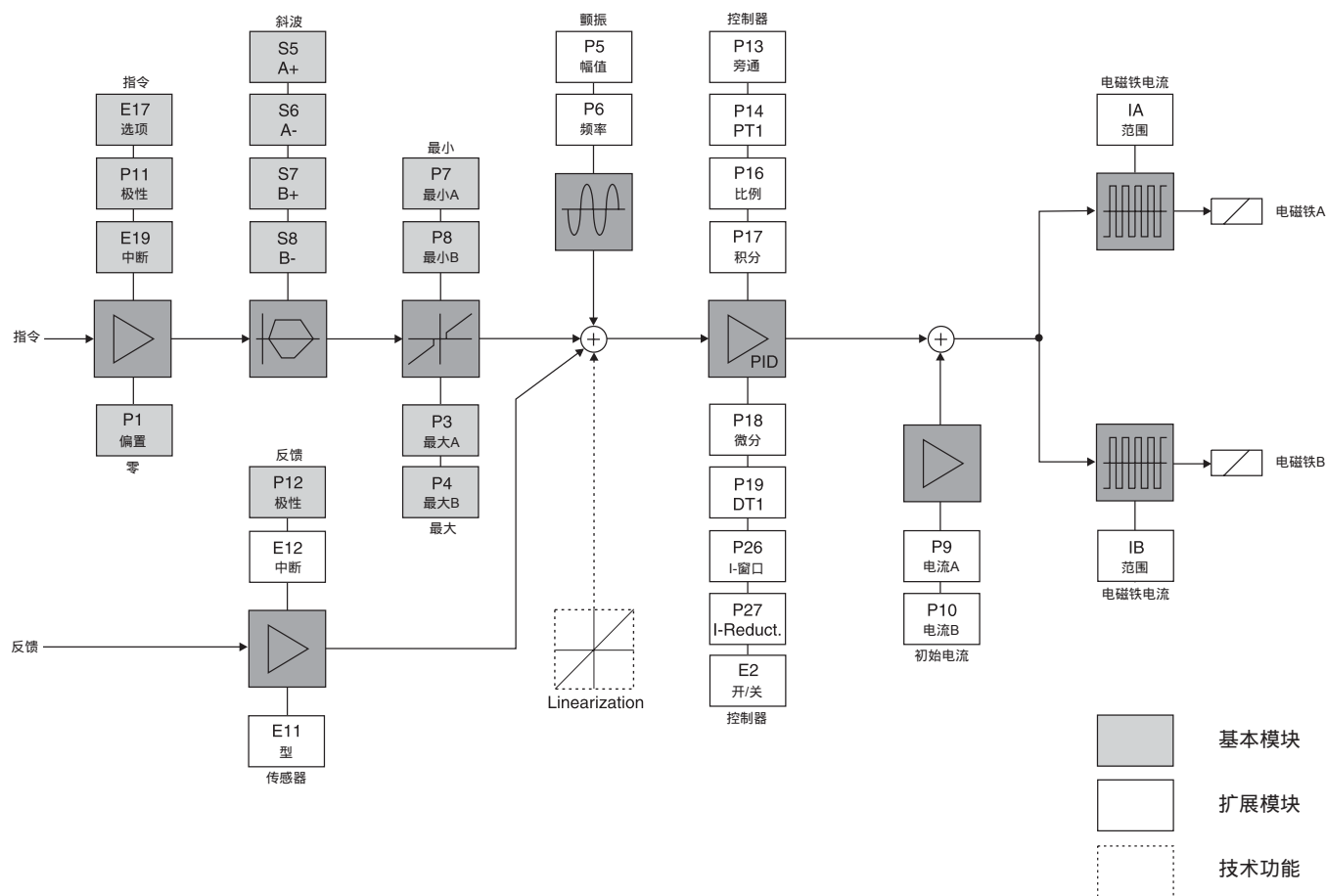
信号流程图
