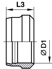
卡套: DPR
