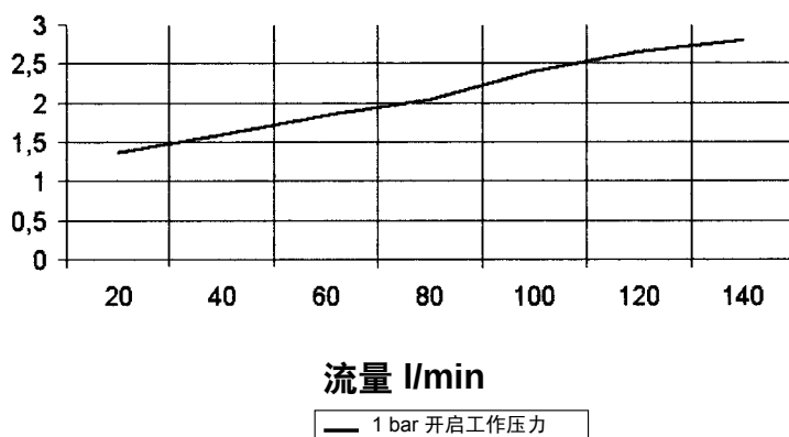
压力降 管外径 28L/30S; 规格16; 英制内螺纹 1 1/4; RVP 47; DN 24
