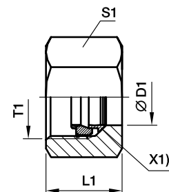
X1) 卡套
