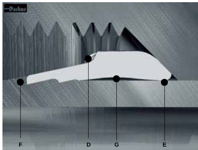
螺母拧紧后
