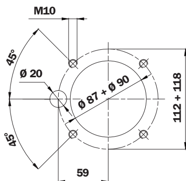
油箱上的孔
