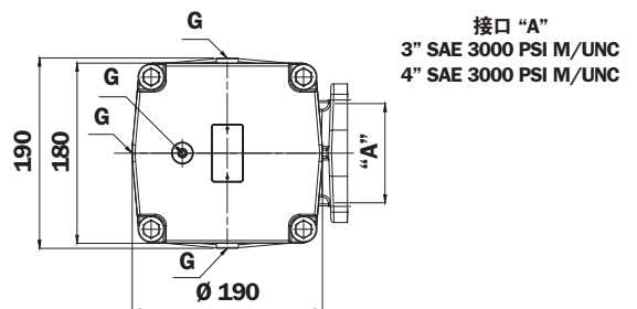
油箱上的孔
