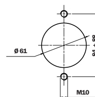
油箱上的孔 MPT 020/021
