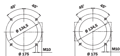
油箱上的孔
