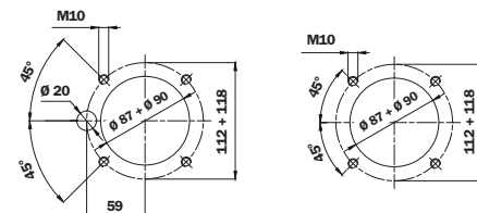
油箱上的孔
