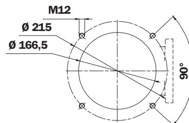
油箱上的孔
