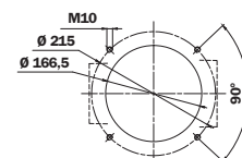
油箱上的孔
