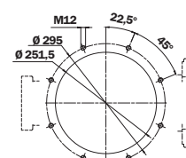
油箱上的孔
