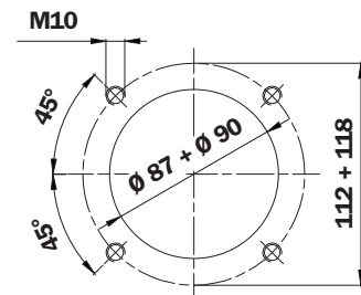
油箱上的孔
