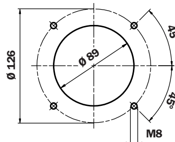
油箱上的孔
