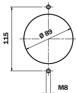
油箱上的孔
