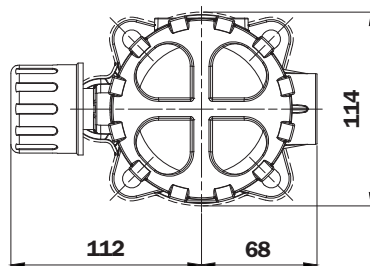
油箱上的孔
