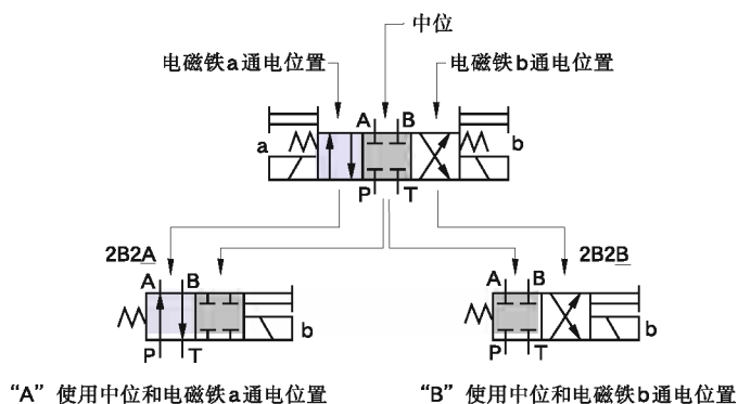
（例）“2”型阀芯
