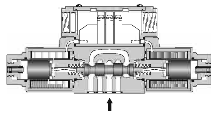
DIN接头型
