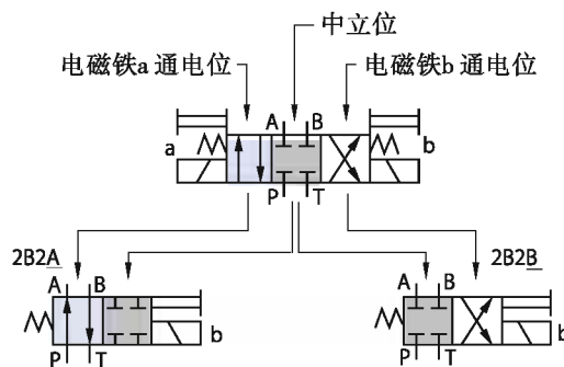
“A” 使用中立位和电磁铁a通电位
